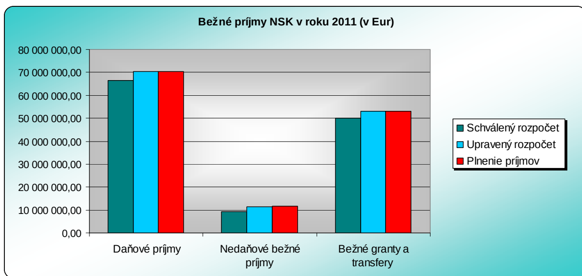
Graf 1: Bežné príjmy NSK v roku 2011
